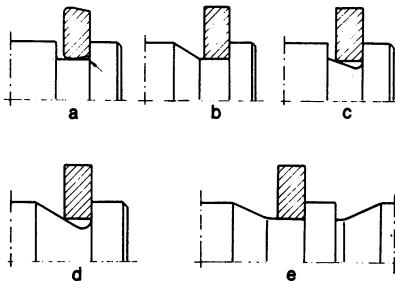
Bild 12: Nutform
